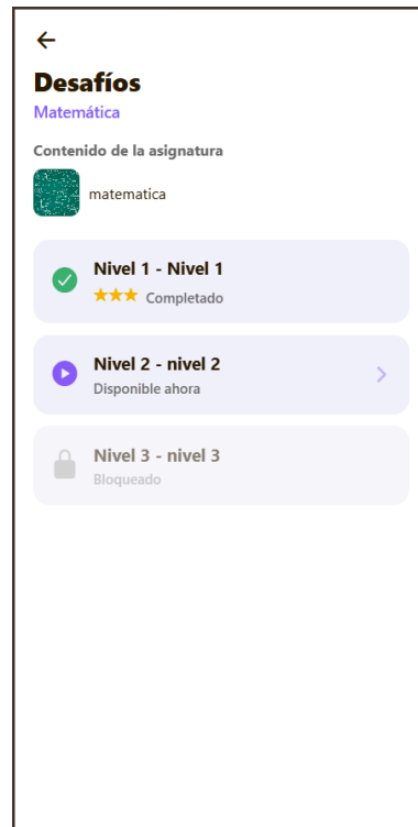
Niveles de la materia Matemática
